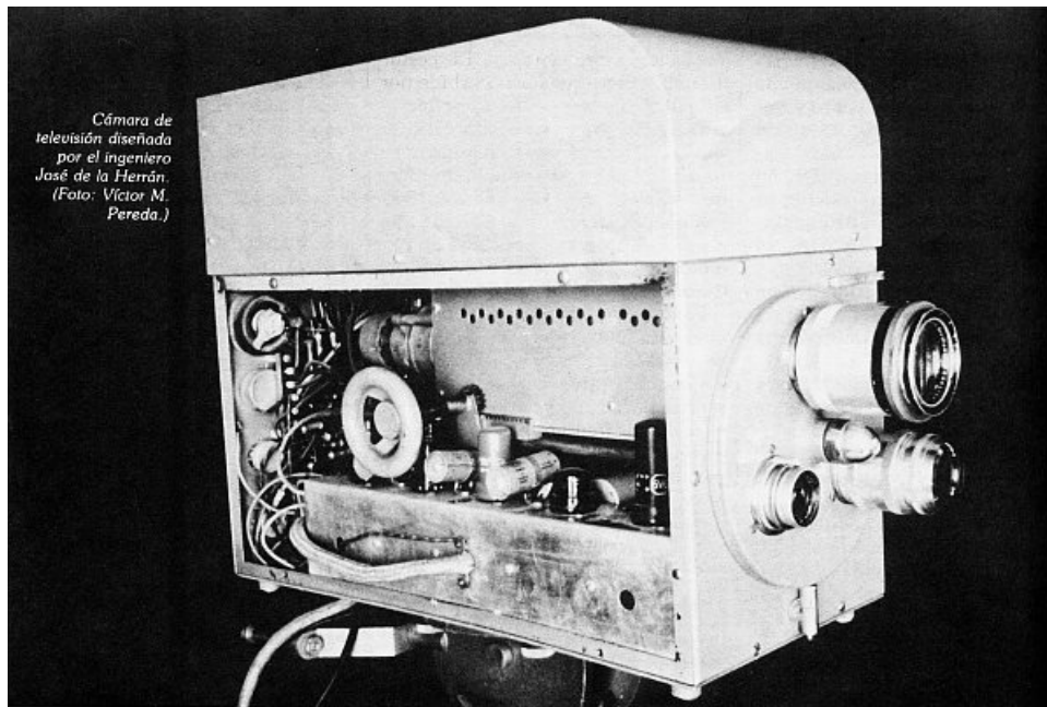
Cámara de televisión diseñada por el ingeniero José de la Herrán. (Foto: Víctor M. Pereda)
