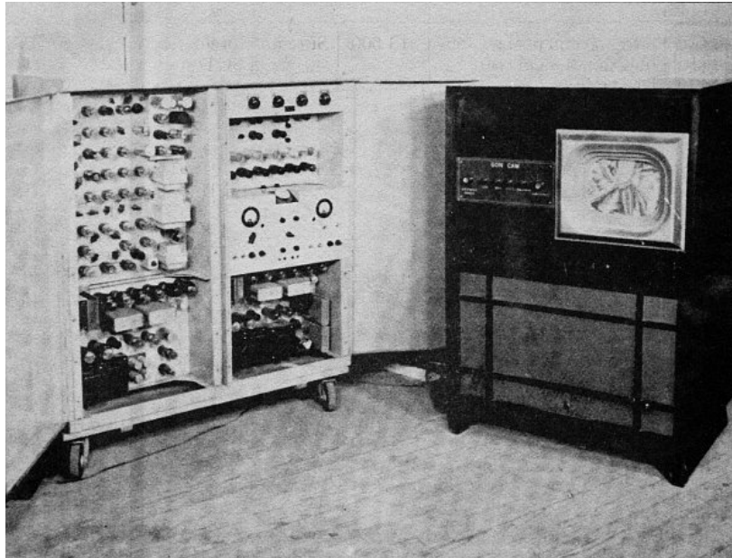
Equipo GON-CAM de televisión a colores que constaba de generar de impulsos, control de cámara y distribuidor de video. (Foto: cortesía de Arturo González Camarena)
