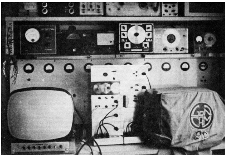
Equipo de televisión en uno de los laboratorios de González Camarena en 1960. (Foto: cortesía de Arturo González Camarena)
